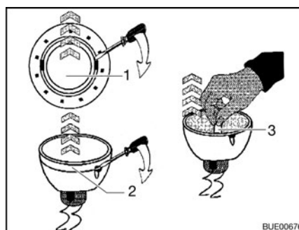
Fig. 235 Cambiar la bombilla halógena
