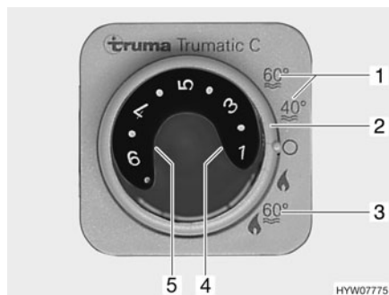
Fig. 169 Unidad de mando para la calefacción/caldera
