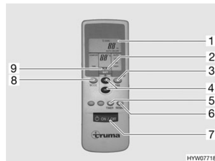
Fig. 165 Mando a distancia
