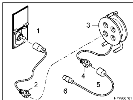
Fig. 133 Posibilidades de conexión de 230 V
