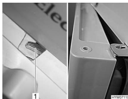
Fig. 188 Puerta del frigorífico/puerta del compartimento congelador en posición de ventilación (Dometic de la serie 7 con compartimento congelador separado)
