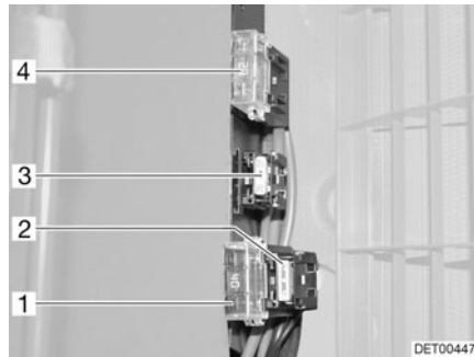
Fig. 139 Fusibles en la batería del habitáculo (Fiat)
