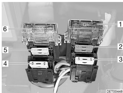
Fig. 136 Fusibles para la batería del motor de arranque (Fiat)
