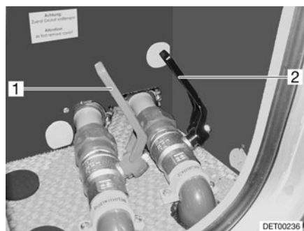
Fig. 199 Grifo para la eliminación de aguas residuales
