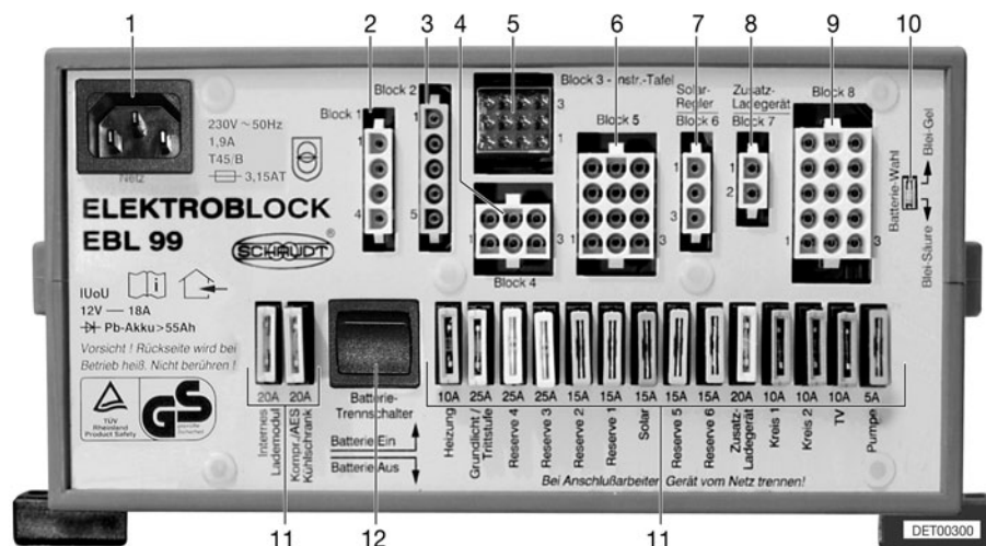
Fig. 127 Bloque eléctrico (EBL 99)
