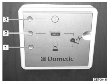
Fig. 213 Panel del inodoro por vacío
