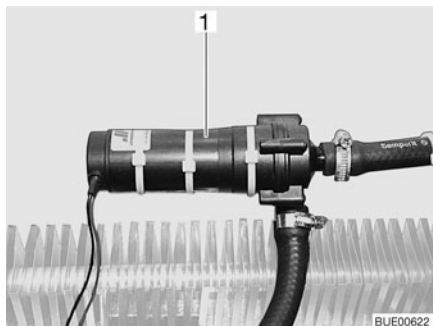
Fig. 155 Bomba de circulación adicional
