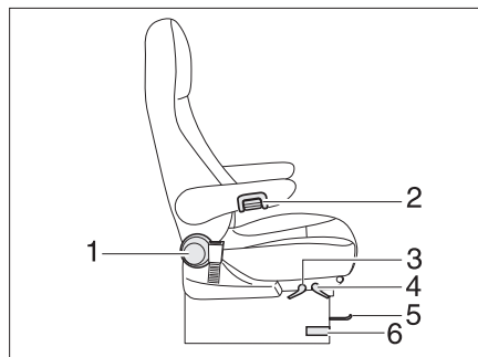
Fig. 13 Asiento del conductor y del acompañante
