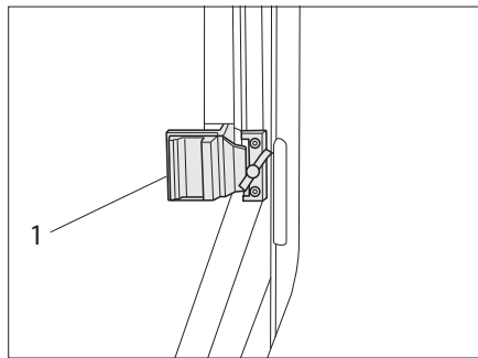
Fig. 48 Ventana corredera con bloqueo corredizo
